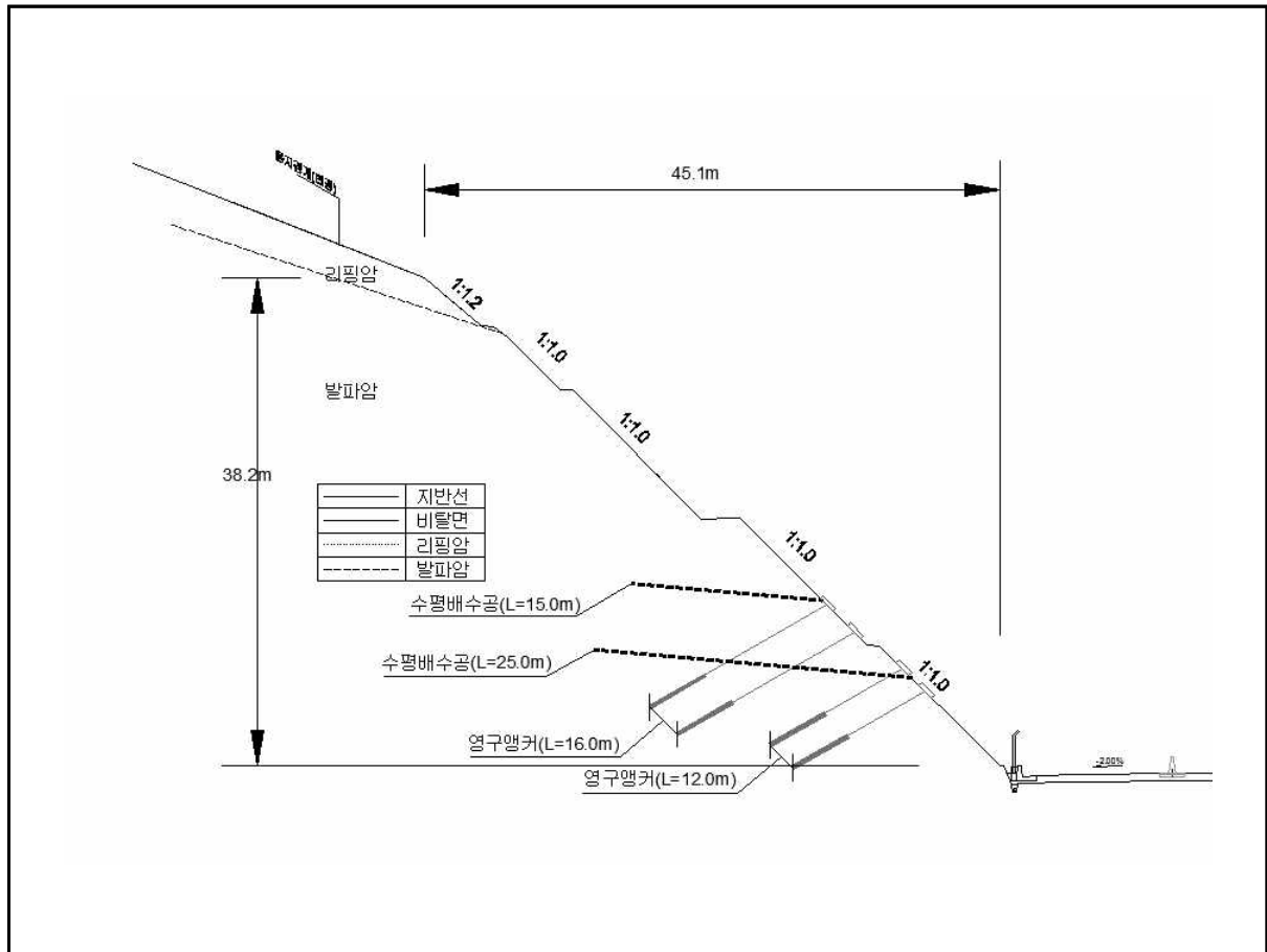
【대표단면 Sta.3+140(상주)】
