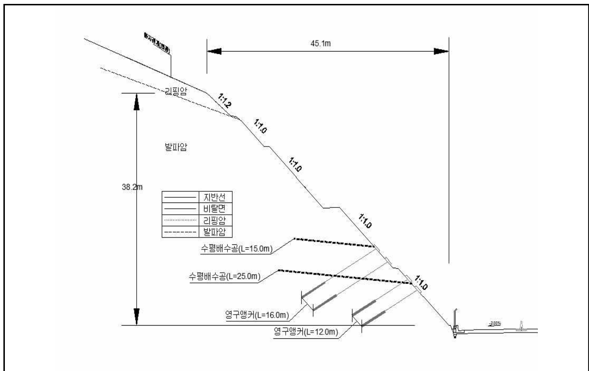
【대표단면 Sta.3+140(영천)】
