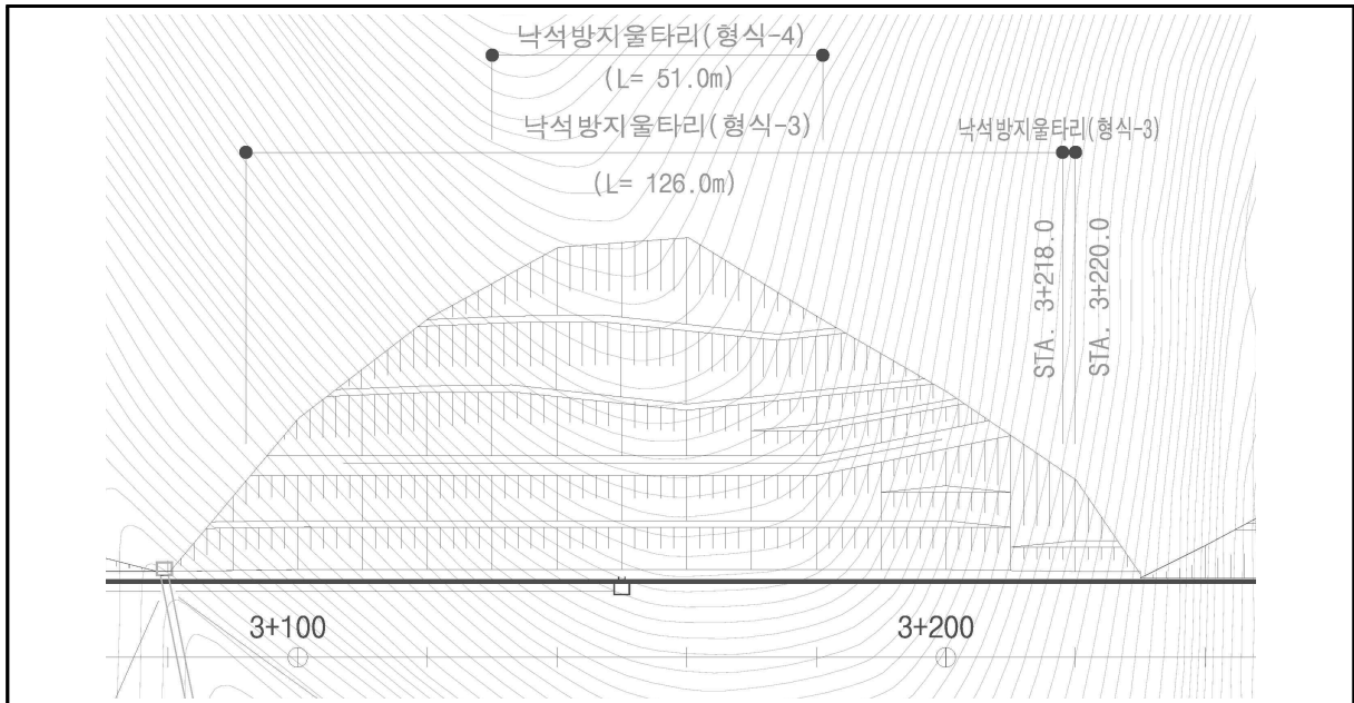
【Sta.3+080~3+240(상주) 평면】
